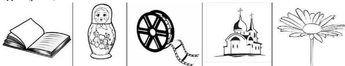
Рис. 1. Примеры картинок
